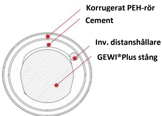
Tvärsnitt av förankringslängden
