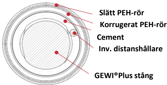
Tvärsnitt av den fria längden
