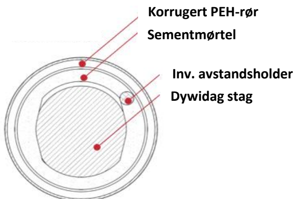
Tverrsnitt av forankringslengden
