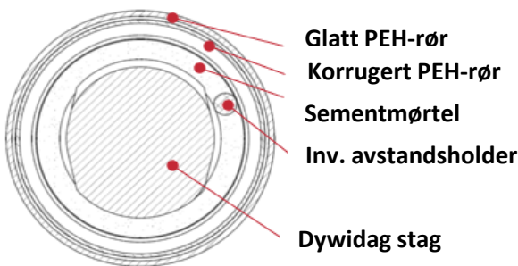
Tverrsnitt av fri lengden
