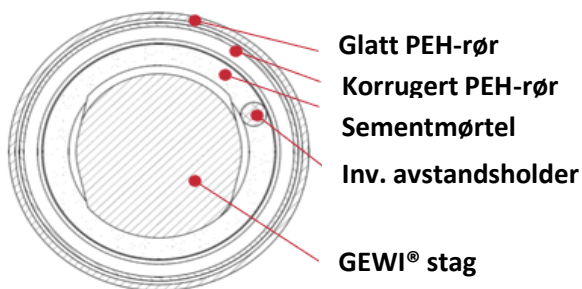
Tversnitt av fri lengden
