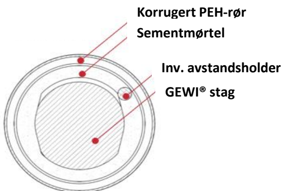
Tversnitt av forankringslengden
